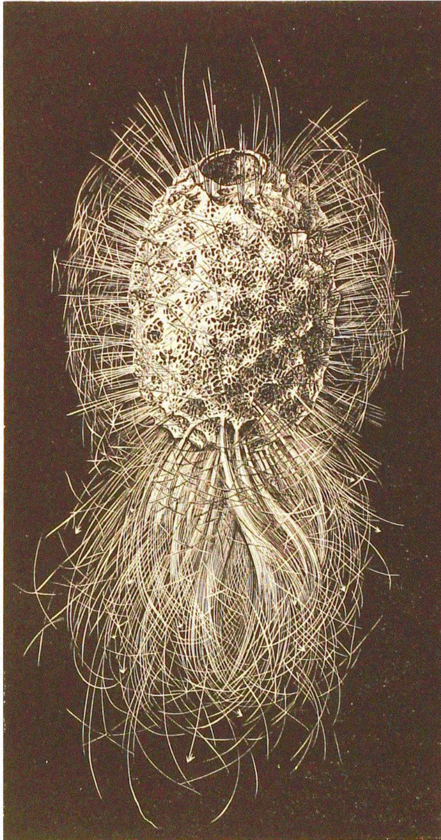
FIG. 65. — Rossella velata , WYVILLE THOMSON. Natural size. (No. 32, 1870.)
